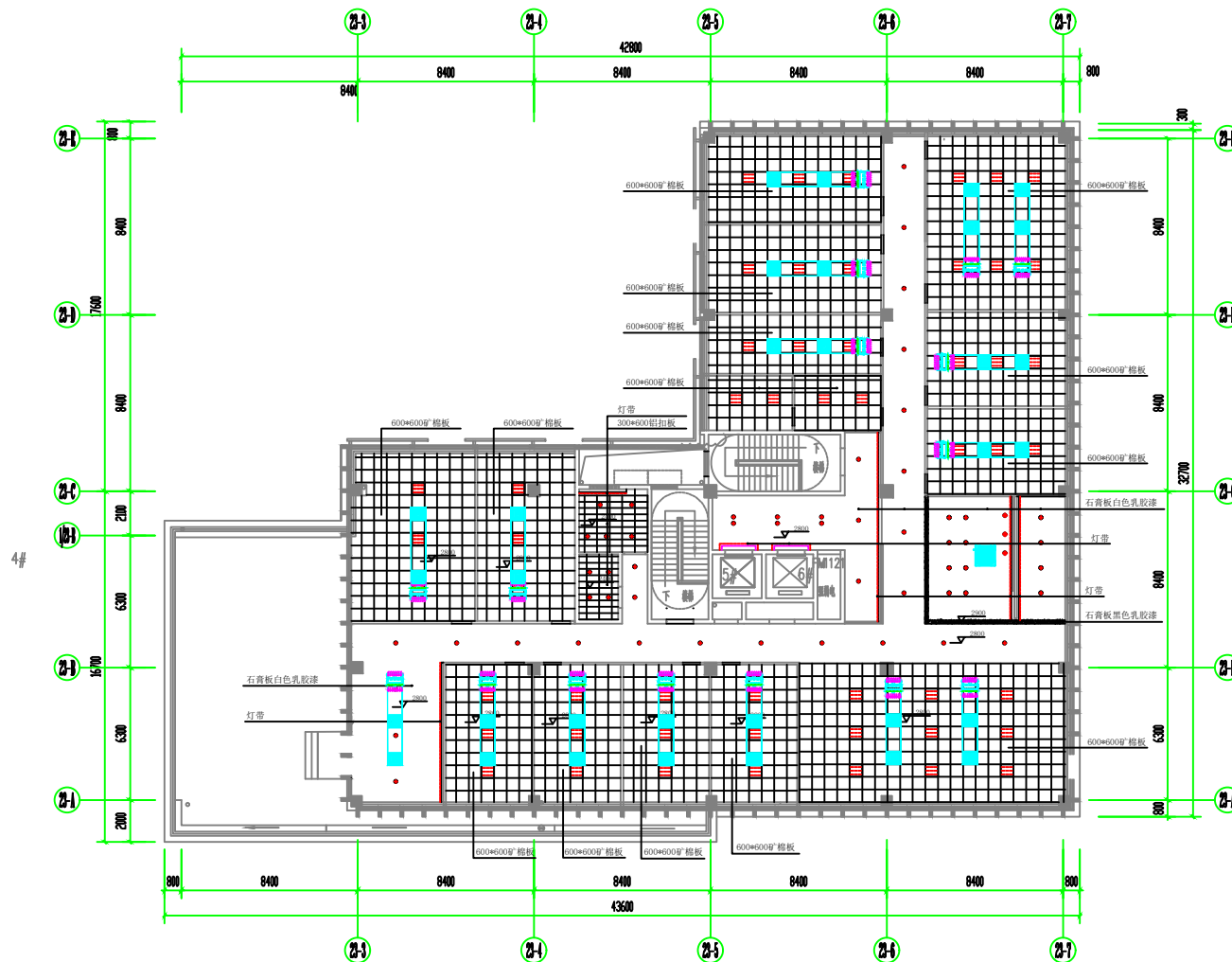
五层空调风管平面图 1:150
